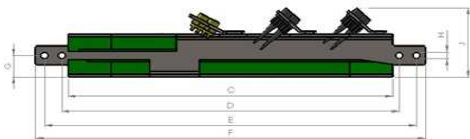
COLLETTORE ASPIRAZIONE A 90°
