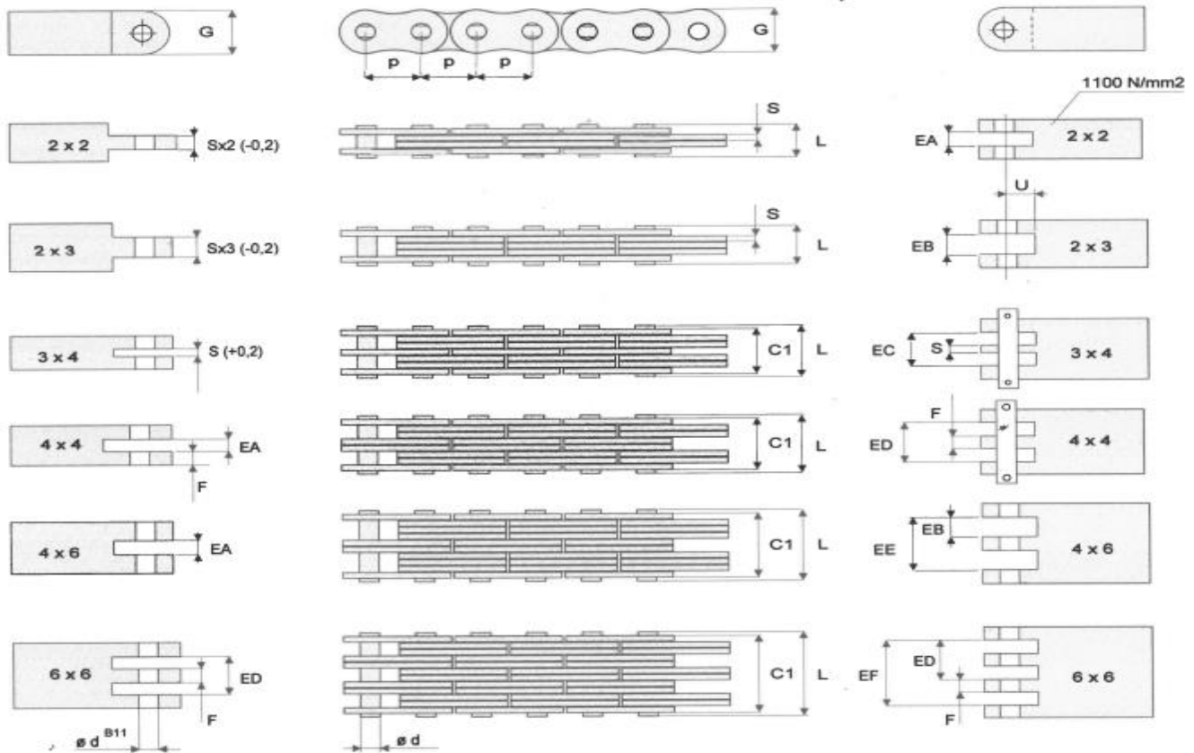
Serie LL DIN 8152-1 (ISO 4347)
