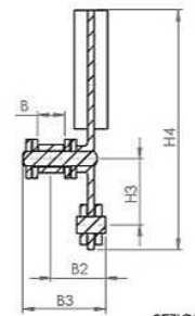
SEZIONE A-A
